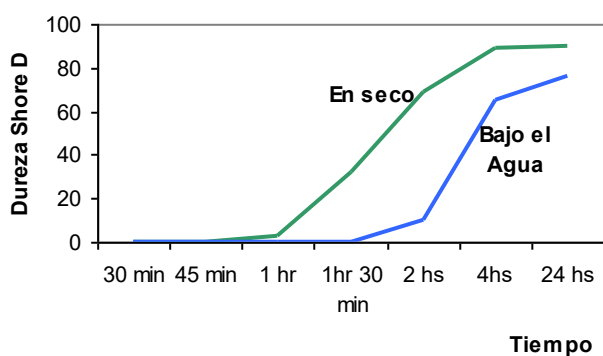
Evolución Dureza Shore D a 15 °C
