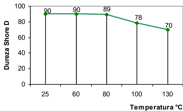
Evolución Dureza Shore D con la Temperatura
