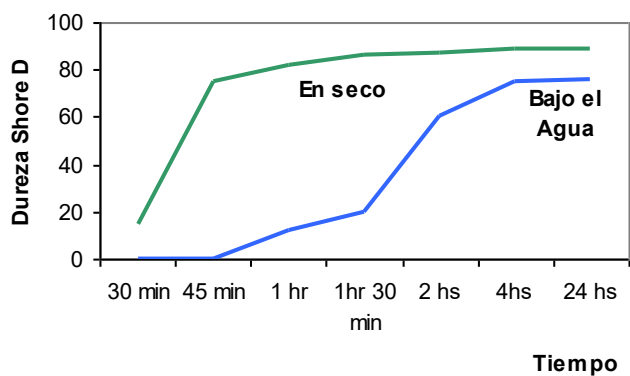
Evolución Dureza Shore D a 35 °C
