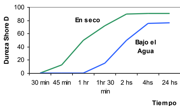
Evolución Dureza Shore D a 25 °C
